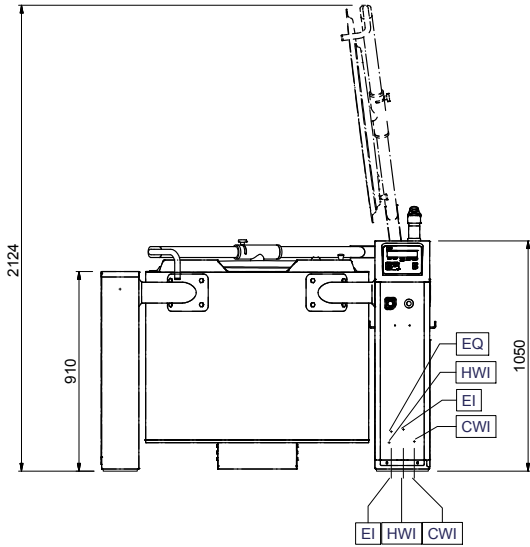
Alzado
